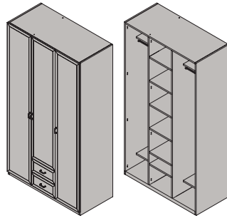
Шкаф 3-дверный ШЗ-02 2130x1257x588 мм
