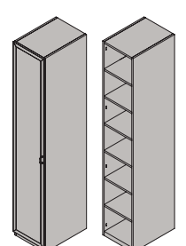
Пенал многоцелевой П1-03 л. 2130x419x588 мм
