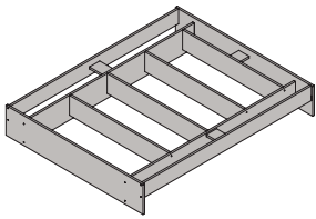
Кровать без спинки КР-01 401x1635x2032 мм (матрас 1600x2000 мм)
