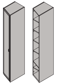
Шкаф переходной ШП-01 л. 2130x405x444/588 мм
