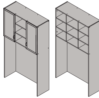
Шкаф-мост ШК-06 2130x1670x444 мм
