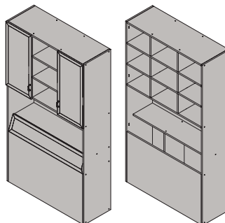
Шкаф прикроватный ШК-03 2130x1270x444 мм
