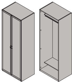
Шкаф 2-дверный для одежды ШЗ-01 2130x838x588 мм
