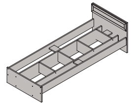
Кровать КР-08 820x870x2032 мм (матрас 800x2000 мм)
