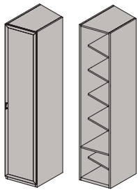
Шкаф переходной ШП-02 п. 2130x405x588/444 мм
