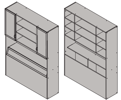
Шкаф прикроватный ШК-01 2130x1670x444 мм
