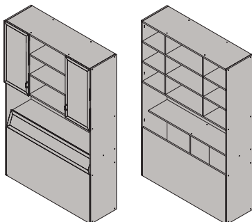
Шкаф прикроватный ШК-02 2130x1470x444 мм
