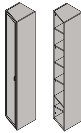
Шкаф переходной ШП-03 л. 2130x405x300/444 мм ШП-05 л. 1800x405x300/444 мм
