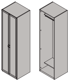
Шкаф 2-дверный для одежды Ш2-21 2130x600x588 мм
