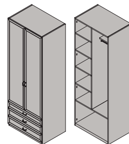
Шкаф 2-дверный универсальный с 3 ящиками ШЗ-09 2130x838x588 мм
