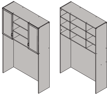
Шкаф-мост ШК-05 2130x1670x444 мм
