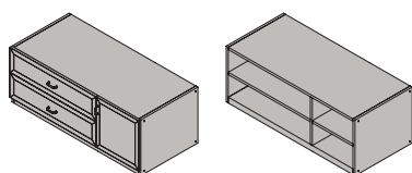
Тумба с 2-ящиками и дверью ТВ-03п. 475x1260x444 мм
