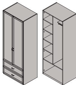
Шкаф 2-дверный универсальный с 2 ящиками ШЗ-06 2130x838x588 мм
