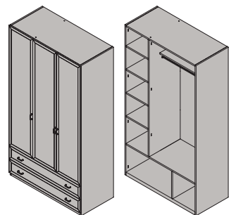
Шкаф 3-дверный ШЗ-04 2130x1257x588 мм
