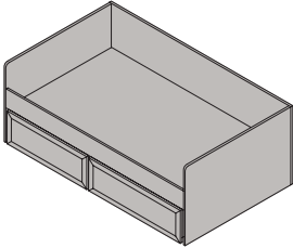
Кровать детская КРД-01 - 715x2035x870 мм (матрас 800x2000 мм) КРД-02 - 715x2035x970 мм (матрас 900x2000 мм)
