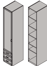
Пенал многоцелевой с 3 ящиками П1-13 л. 2130x419x444 мм
