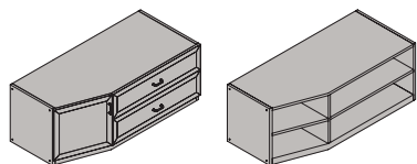
Тумба с 2-ящиками и дверью ТВ-01 л. 475x1260x444/588 мм
