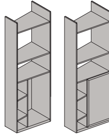
Шкаф-стеллаж со скосной дверью СТД-01 левый 2130x620x270/444 мм
