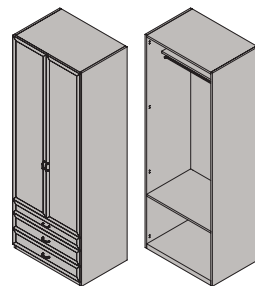
Шкаф 2-дверный для одежды с 3 ящиками ШЗ-07 2130x838x588 мм
