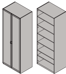
Шкаф 2-дверный многоцелевой ШЗ-02 2130x838x588 мм
