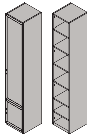
Пенал многоцелевой с 2 дверьми П1-18 п. 2130x419x444 мм П1-26 п. 1800x419x444 мм
