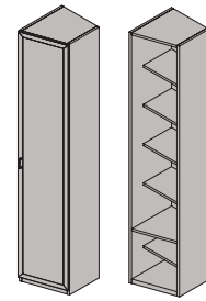
Шкаф переходной ШП-04 п. 2130x405x444/300 мм ШП-06 п. 1800x405x444/300 мм
