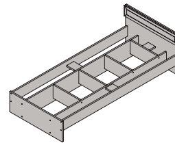
Кровать КР-07 820x970x2032 мм (матрас 900x2000 мм)
