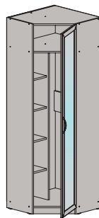
Шкаф угловой 2130x730/742x444 мм
