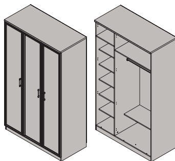
Шкаф 3-х дверный ФШ3-01 2330x1257x599 мм
