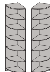
Стеллаж с полукругами ФСТ1- 2330x454x454 мм ФСТ2- 2330x599x599 мм ФСТ3- 2330x454/599x599/454 мм ФСТ4- 1830x454x454 мм
