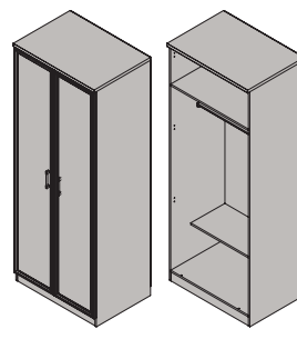
Шкаф 2-х дверный ФШ2-01 2330x838x599 мм
