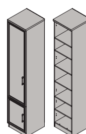
Пенал многоцелевой с 2 дверьми ФП1-17 левый ФП1-25 левый 2330x419x599 мм 1830x419x454 мм
