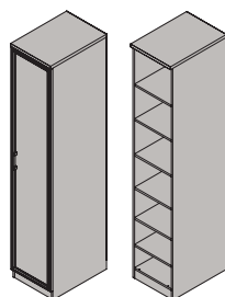
Пенал многоцелевой ФП1-04 правый 2330x419x599 мм
