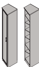
Шкаф переходной ФШП-03 левый ФШП-05 левый 2330x405x310/454 мм 1830x405x310x454 мм
