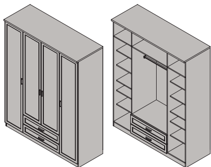
Шкаф 4-х дверный с 2 ящиками ФШ4-01 2330x1680x599 мм
