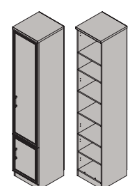
Пенал многоцелевой с 2 дверьми ФП1-17 правый ФП1-26 правый 2330x419x599 мм 1830x419x454 мм
