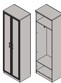
Шкаф 2-дверный с выдвижной штангой ФШ2-22 2330x600x454 мм
