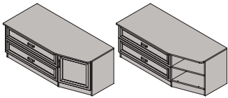
Тумба ТВ с 2 ящиками и дверью ФТВ-01 правая 475x1260x599/454 мм
