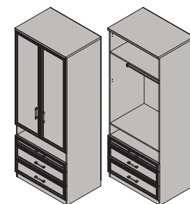
Шкаф 2-х дверный, с нишей и 3 ящиками ФШ2-10 2330x838x599 мм
