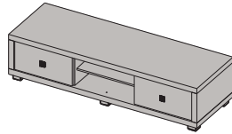
ОТВ-02 Тумба ТВ с 2 ящиками и нишей 431x1782x596 мм
