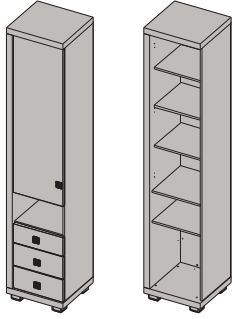
ОП1-01 Пенал многоцелевой с дверью, 3 ящиками и нишей (левый) 2284x473x452 мм
