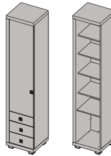
ОП1-07 Пенал многоцелевой с дверью, 3 ящиками (левый) 2284x473x452 мм
