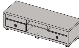
ОТВ-03 Тумба ТВ с 2 ящиками и нишами 492x1782x596 мм
