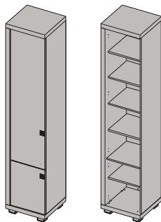
ОП1-13 Пенал многоцелевой 2-дверный (левый) 2284x473x452 мм
