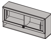
ОПБ-08 Полка-бар 1-дверная (стекло) с нишей 573x1198x309 мм
